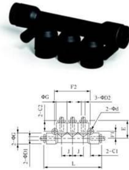
PK 系列 五通接管 PK Series Triple branch
