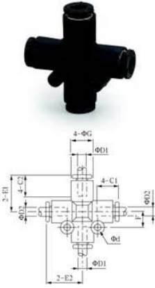
PZA 系列 四通接管 PZA Series Union cross
